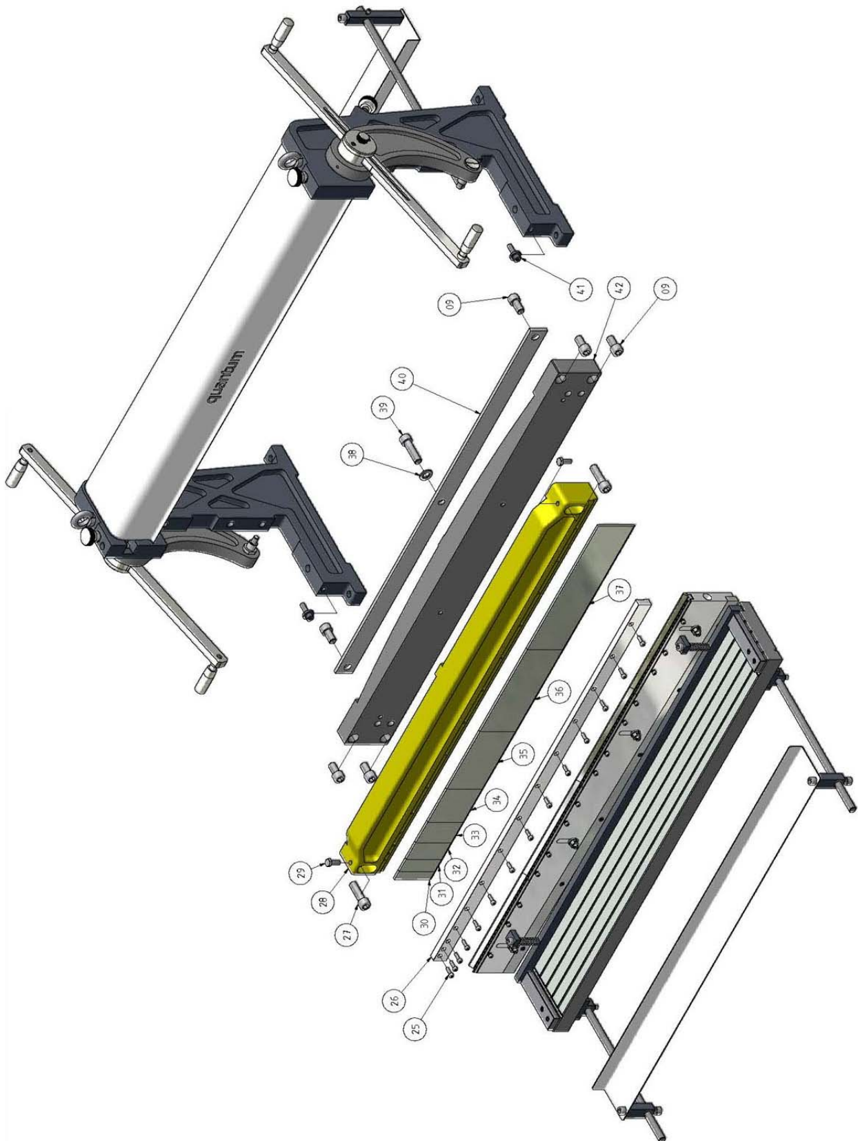
Abb.6-2: Ersatzteilzeichnung 2-4 - Drawing spare parts 2-4
